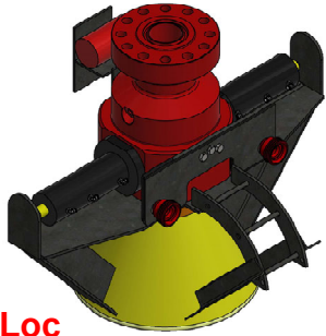
RamLoc Tool
